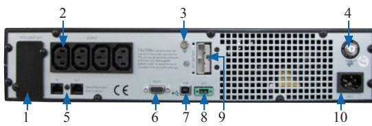
Réf. 30005 (2kVA, 2U, PROF. 654mm)
