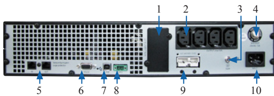
Réf. 30013 (4kVA, 2U, prof. 454mm)
