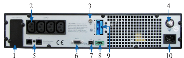
Réf. 30006 (3kVA, 2U, prof. 654mm)
