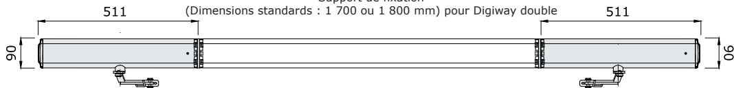
Digisimple double avec bras universel (Tirant/Poussant) en mode articulé + profilé central
