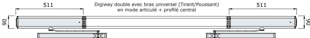
Digisimple double avec bras universel (Tirant/Poussant) en mode coulissant + profilé central
