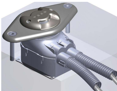
Boîte d'encastrement (6009612) + Plaque (6011309)
